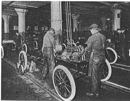
El comienzo de la producción en masa (1913). En los primeros trenes de montaje, el chasis se empujaba a mano.
